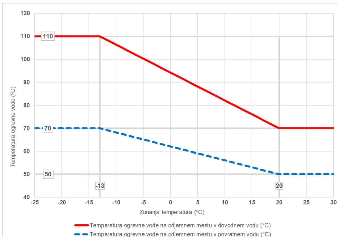
Diagram 4: Temperaturni diagram za zunanjo normno temperaturo -13°C (2C toplovodni sistem 110/70°C, NP 16)
