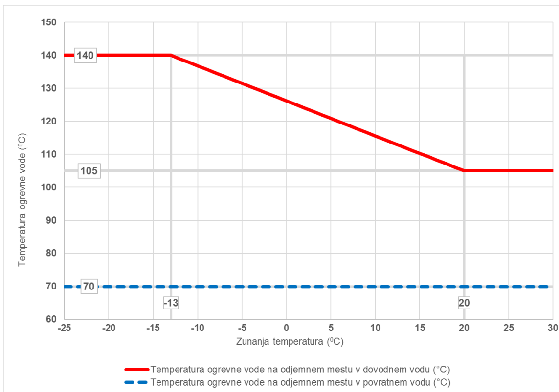
Diagram 2: Temperaturni diagram za zunanjo normno temperaturo -13°C (2C vročevodni sistem 140/70°C, NP 16 ali NP 25)
