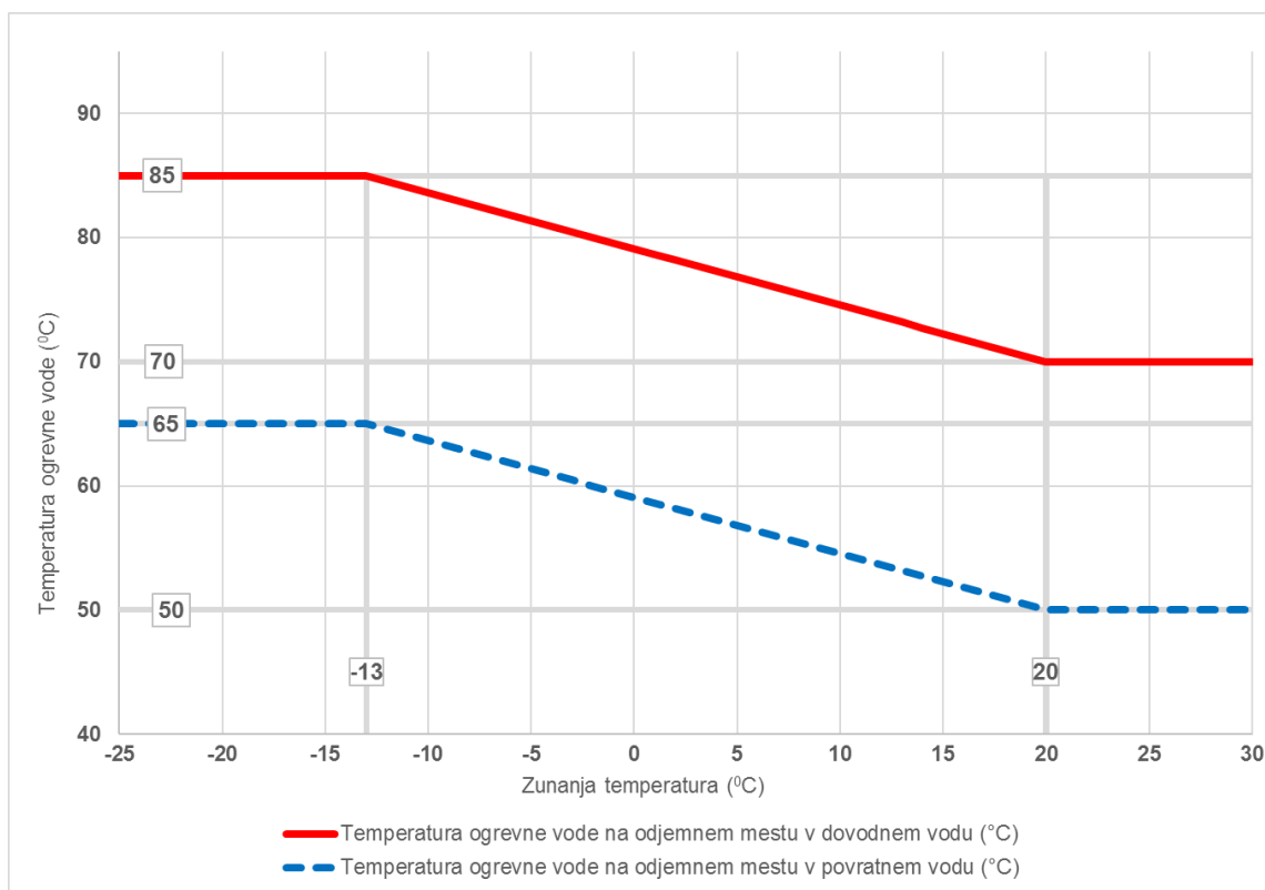
Diagram 5: Temperaturni diagram za zunanjo normno temperaturo -13°C (4C toplovodni sistem 85/65°C, NP 6)
