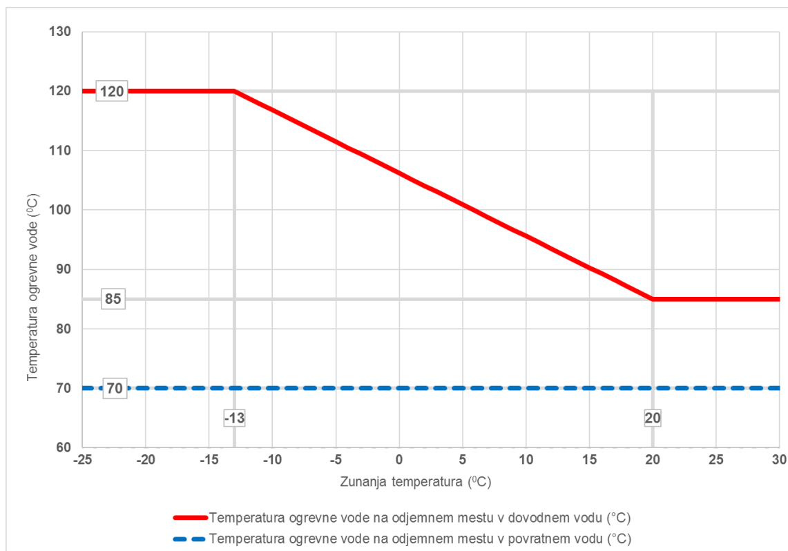
Diagram 3: Temperaturni diagram za zunanjo normno temperaturo -13°C (2C toplovodni sistem 120/70°C, NP 16)
