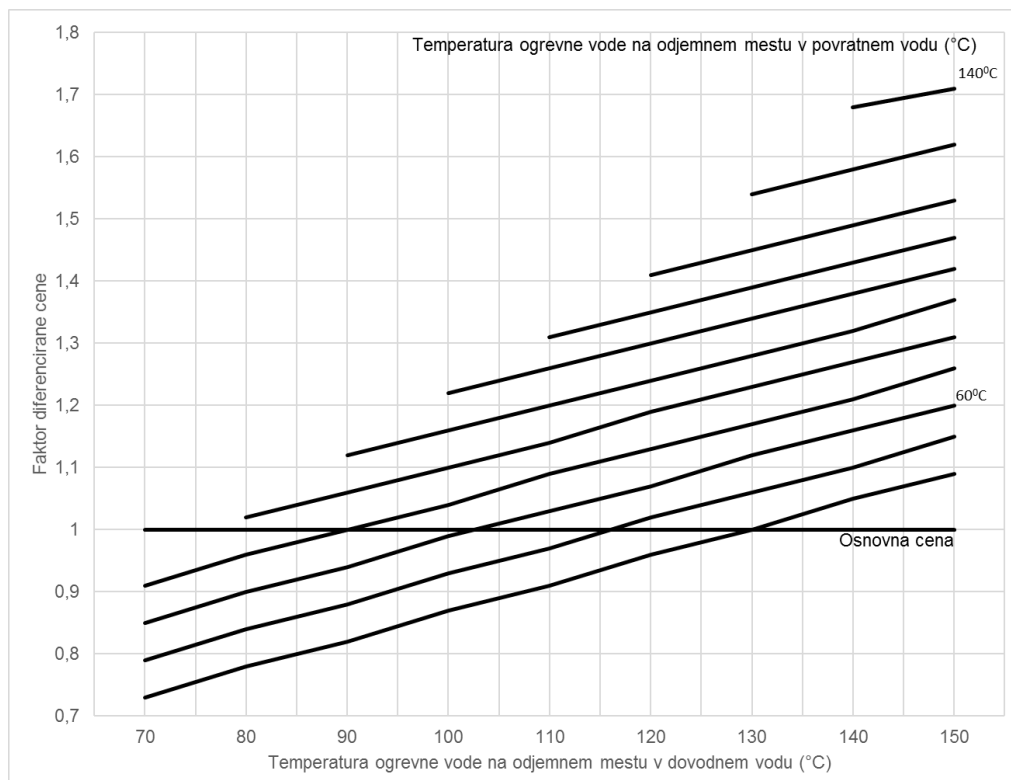
Diagram 1: Diagram za določitev faktorja diferencirane cene toplote
