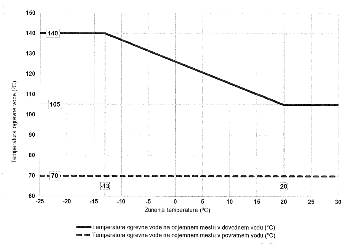
Diagram 1 Vročevodni (2C) sistem daljinskega ogrevanja z ogrevnim medijem vročo vodo, nazivna temperatura 140 °C
